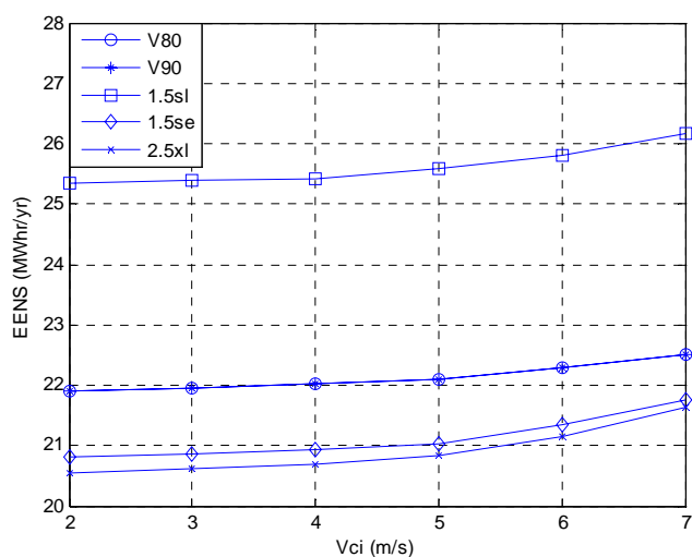
Fig. 9 EENS versus wind turbine cut-in speed
